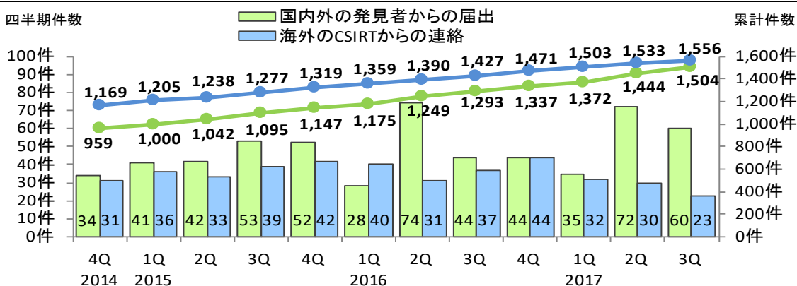
図 2-11. ソフトウェア製品の脆弱性対策情報の公表件数
