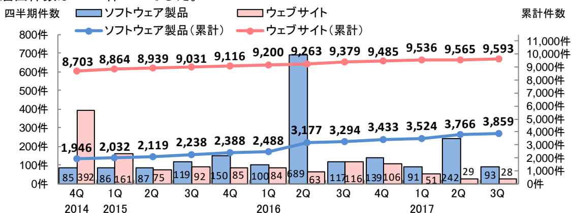
図 1-1. 脆弱性の届出件数の四半期ごとの推移
